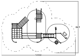
LAPPSET Q16556 EN Impact Area 23,5 m 2 EN Falling Space 72,8 m 2
