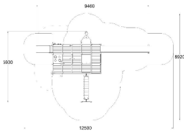
LAPPSET. Q16178 EN Impact Area 61.0 m 2 EN Falling Space 65.9 m 2
