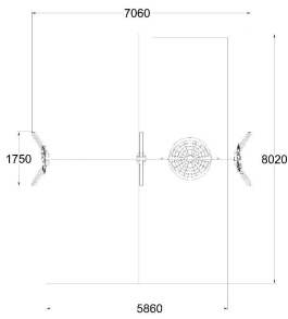
LAPPSET. Q15813 EN Impact Area 43.1 m 2 EN Falling Space 43.1 m 2
