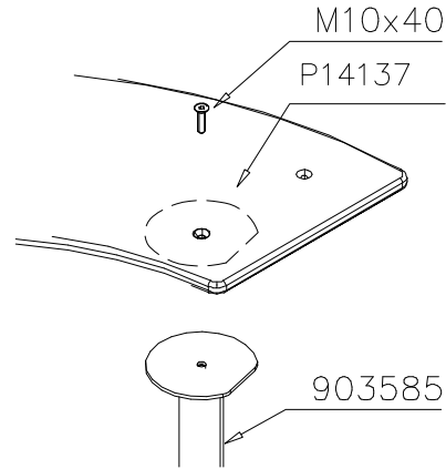
DET 2
