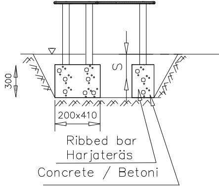
DET 1
