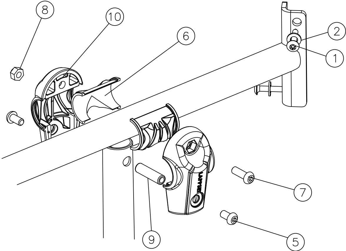
DET 1
