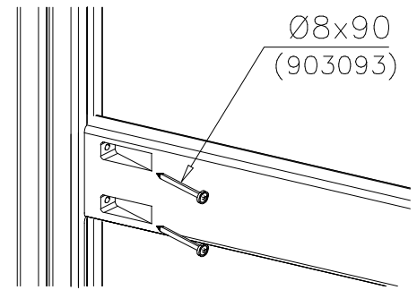
DET 3
