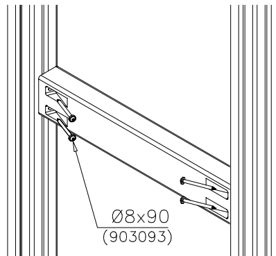
DET 5
