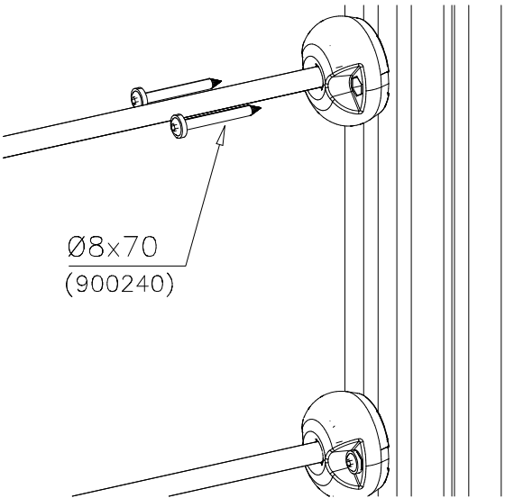
DET 22
