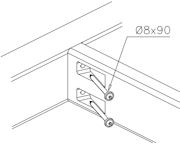
DET 27
