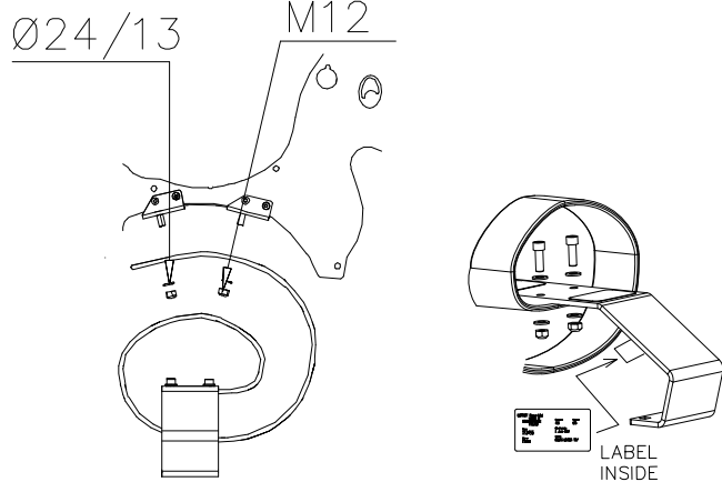
DET 5
