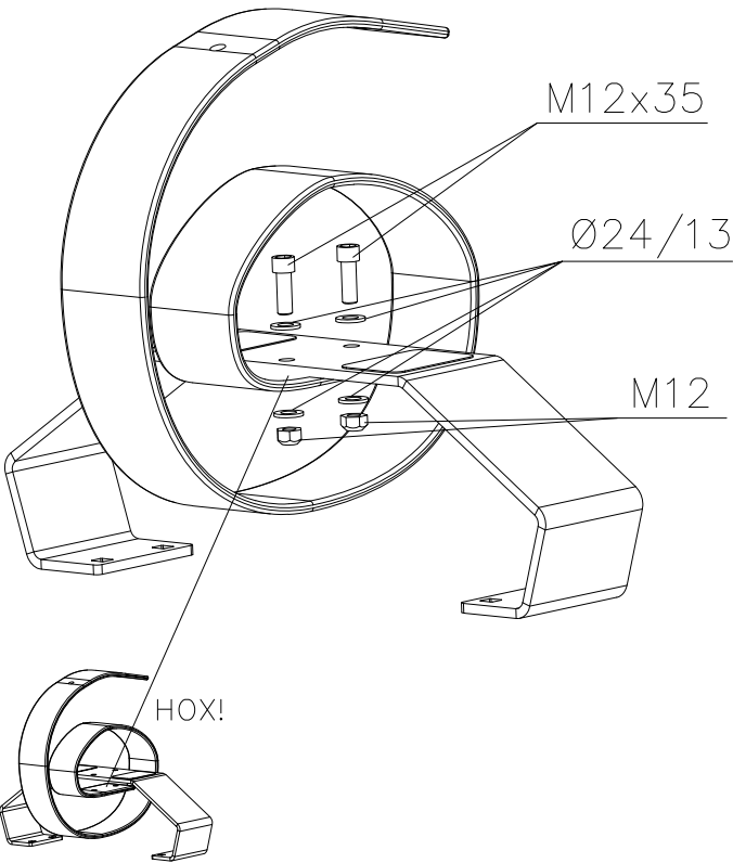
DET 4
