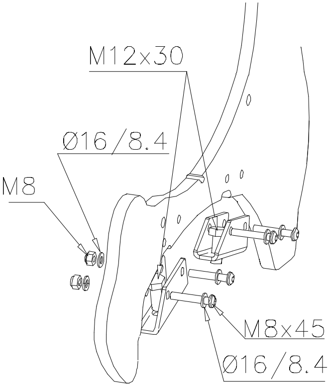
DET 1
