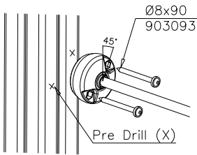
DET 2
