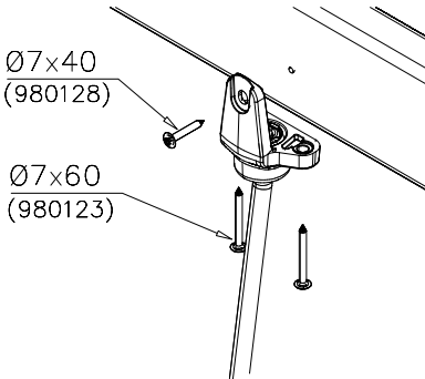
DET 2
