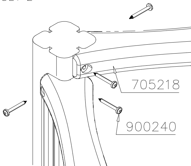
DET 2
