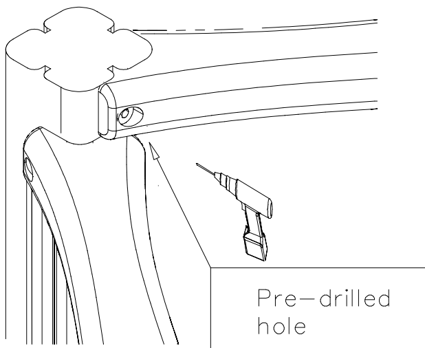
DET 1
