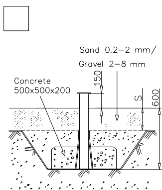
DET 4
