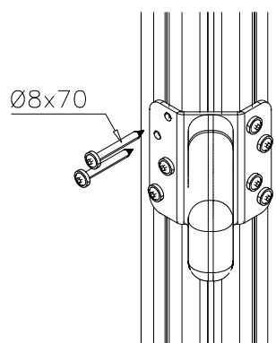
DET 5
