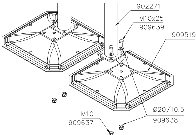
DET 4
