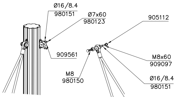
DET 8
