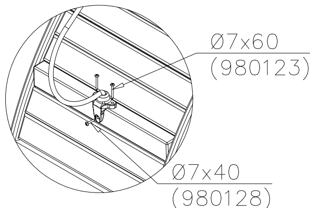
DET 6
