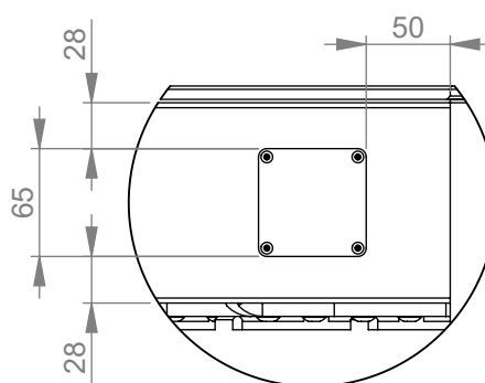
DETAIL A 1 : 5
