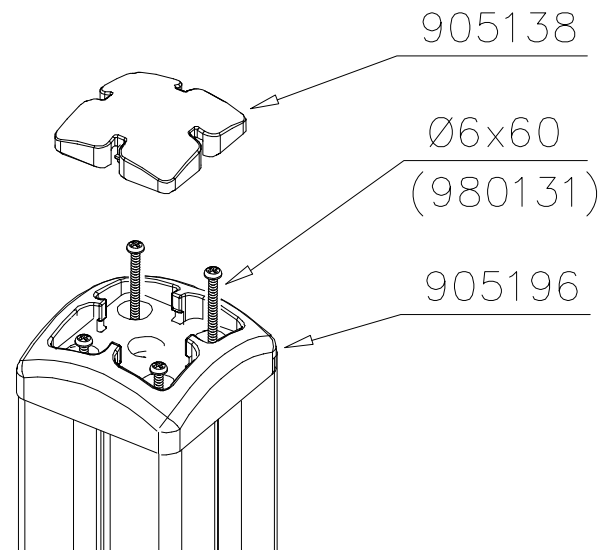
DET 10
