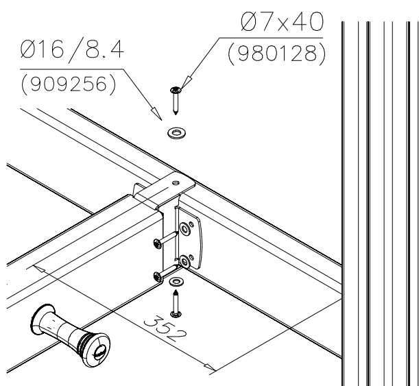
DET 3
