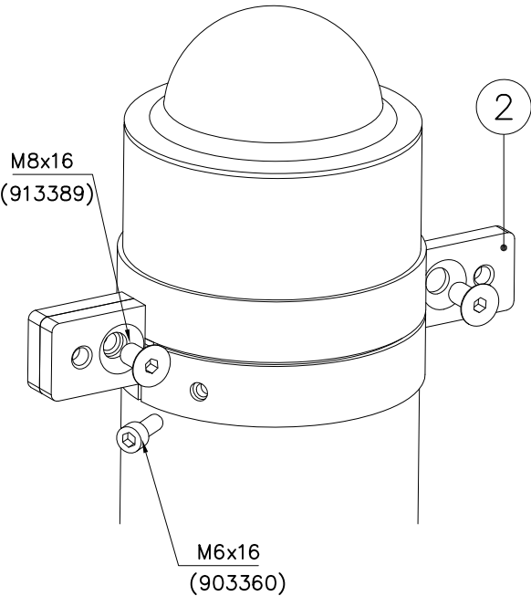
DET 1
