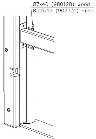
DET 3
