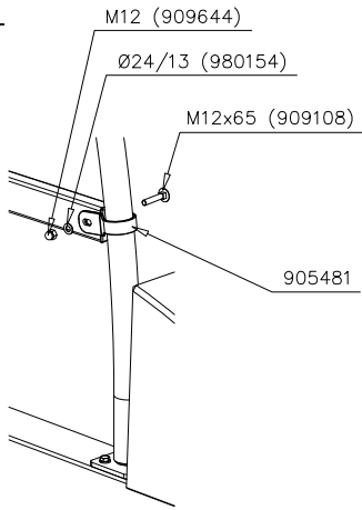
DET 4
