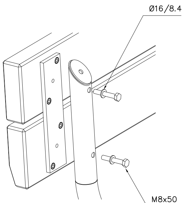
DET 2
