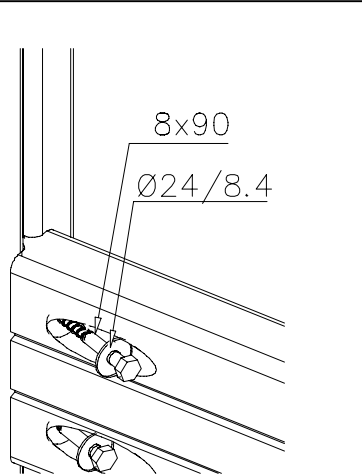
DET 1
