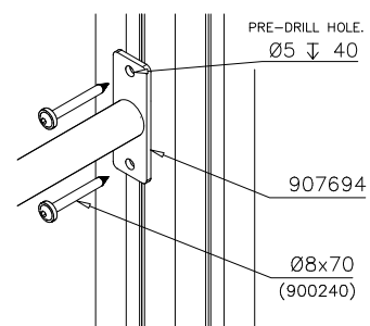
DET 1
