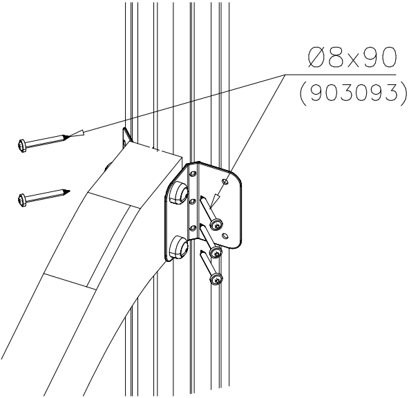
DET 3
