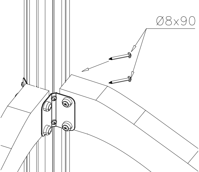
DET 6
