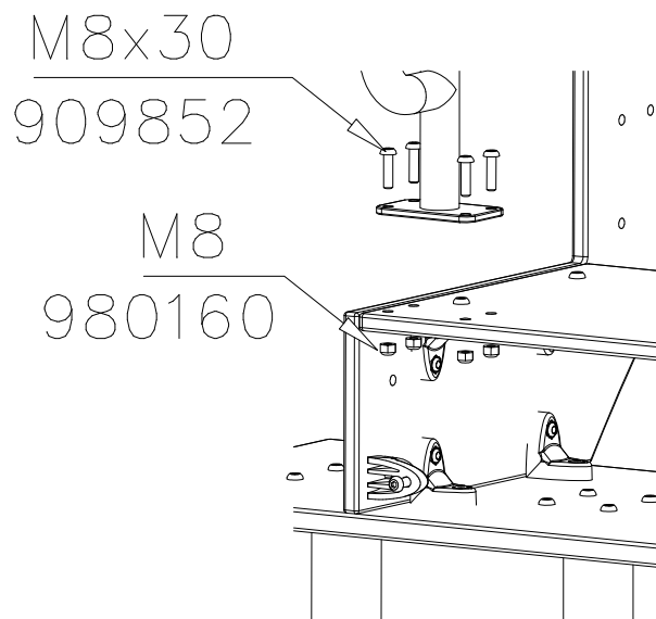
DET 19
