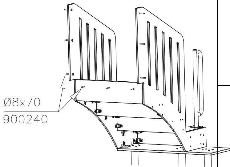
DET 20
