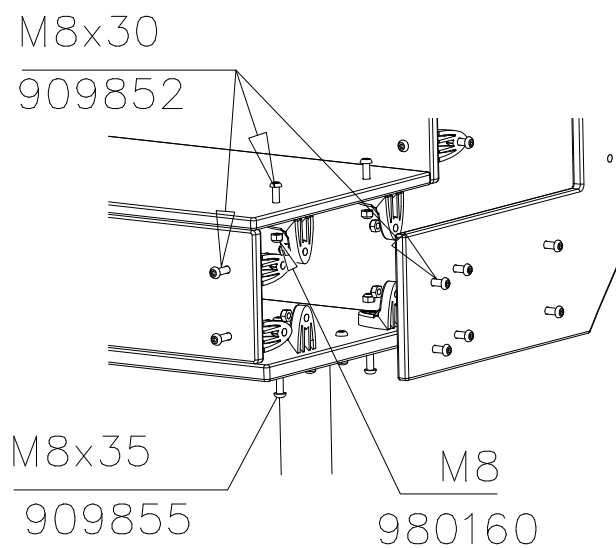
DET 18
