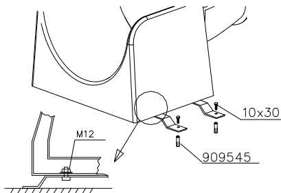
DET 11
