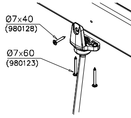
DET 22
