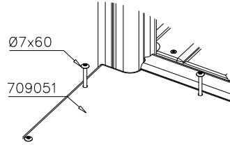
DET 23
