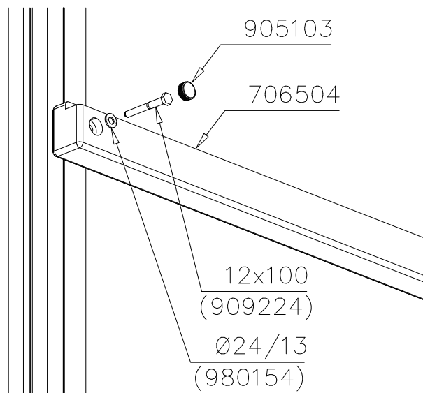
DET 9
