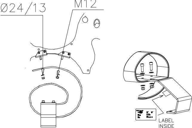
DET 5
