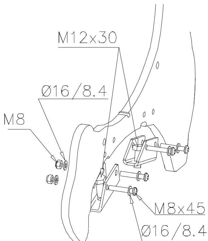
DET 1
