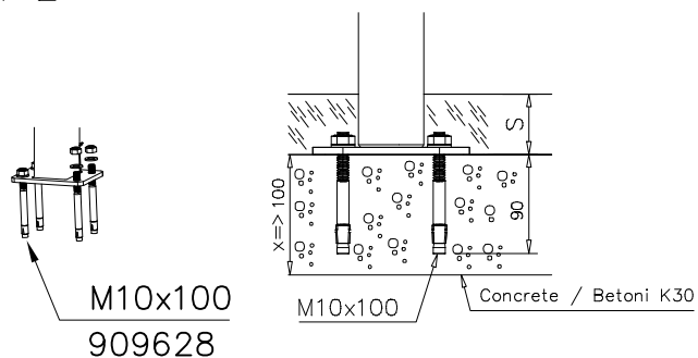
DET 2
