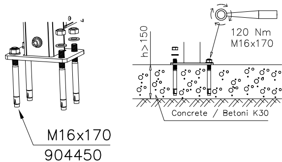
DET 1
