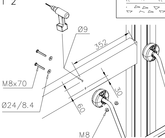
DET 2
