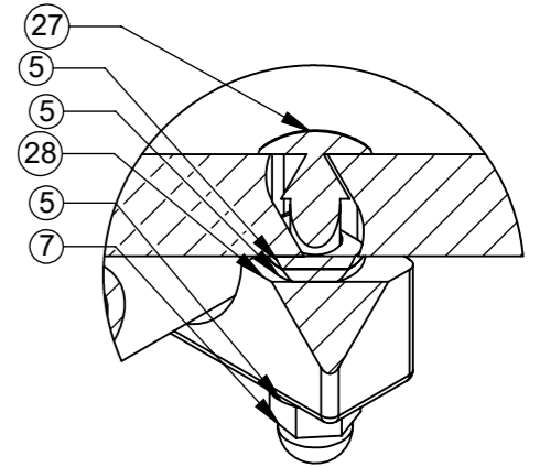
DETAIL B 1 : 2
