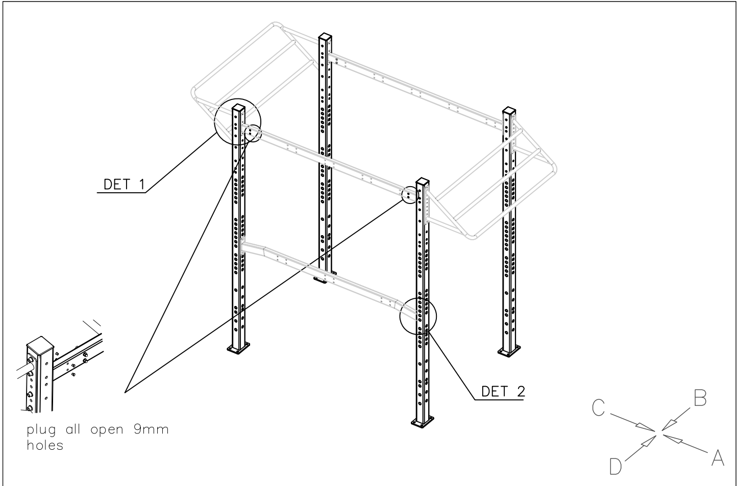
DET 1
