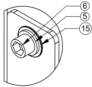
DETAIL D 1 : 2
