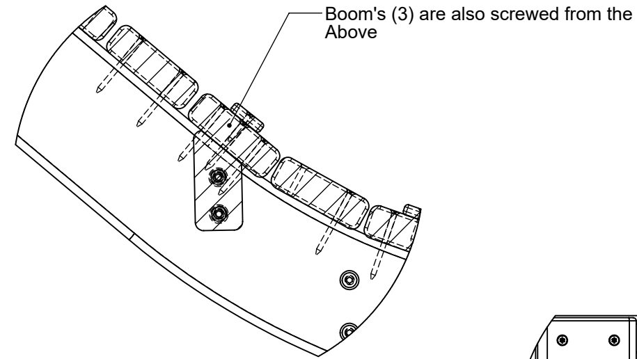
DETAIL H 1 : 5
