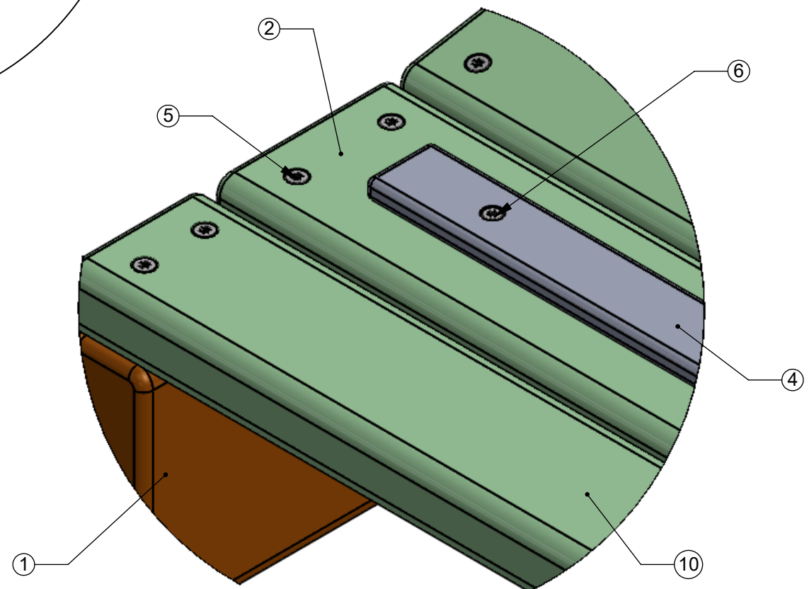
DETAIL A 1 : 2
