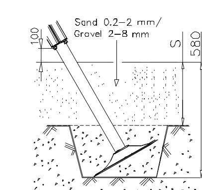
DET 2
