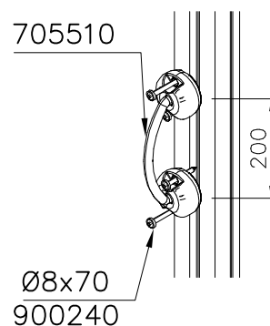
DET 6
