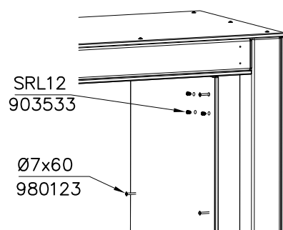
DET 7
