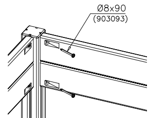
DET 1
