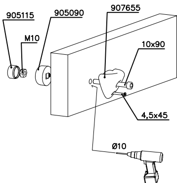
DET 4
