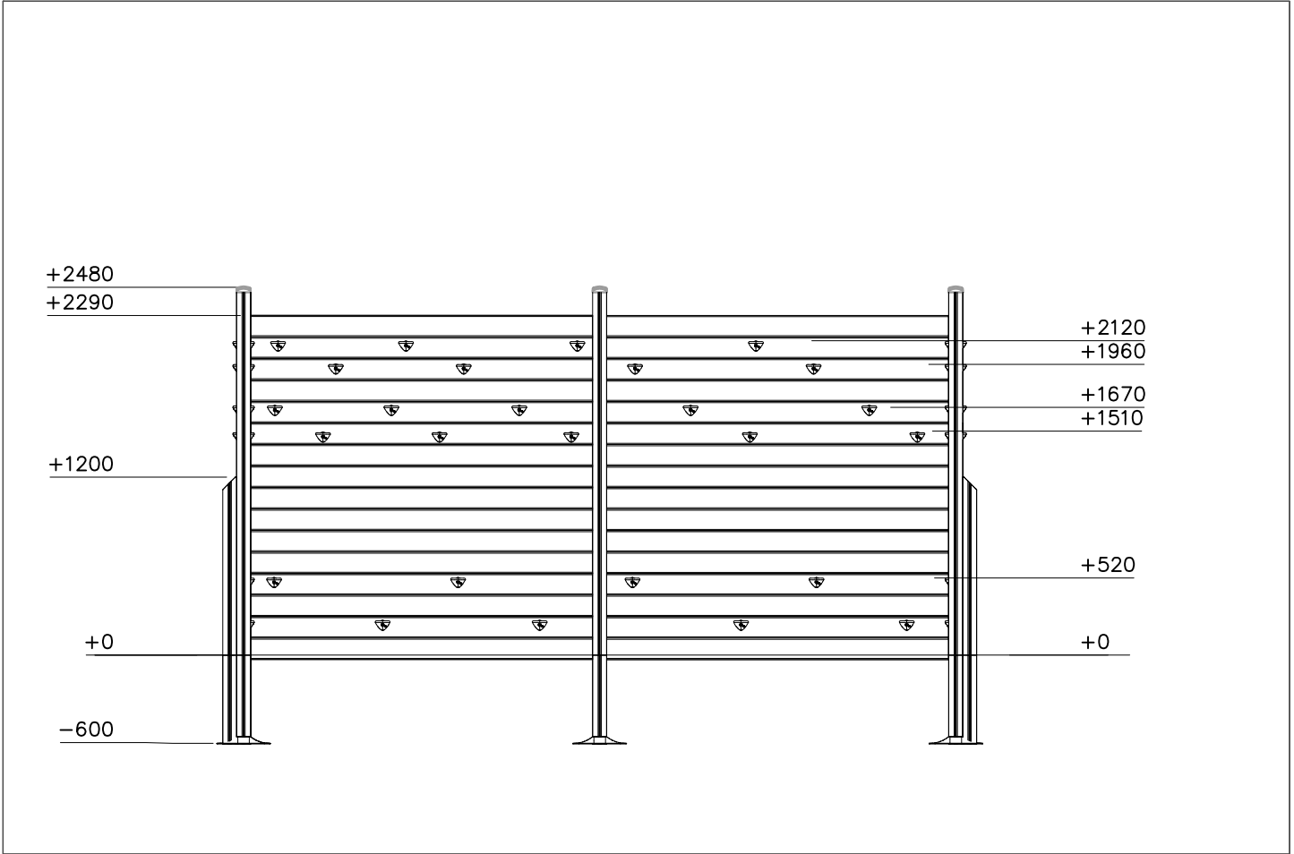
DET 1
