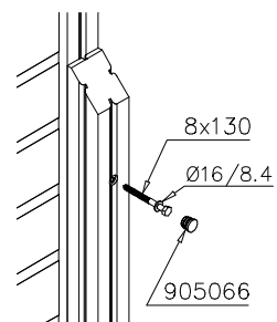
DET 3
