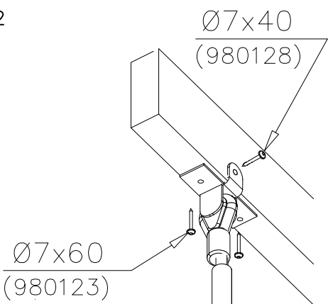
DET 2
