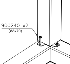
DET 28
