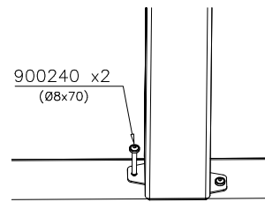
DET 24
