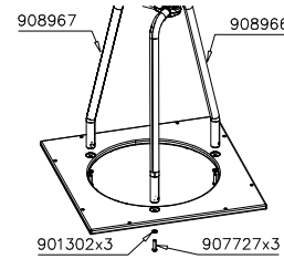
DET 32
