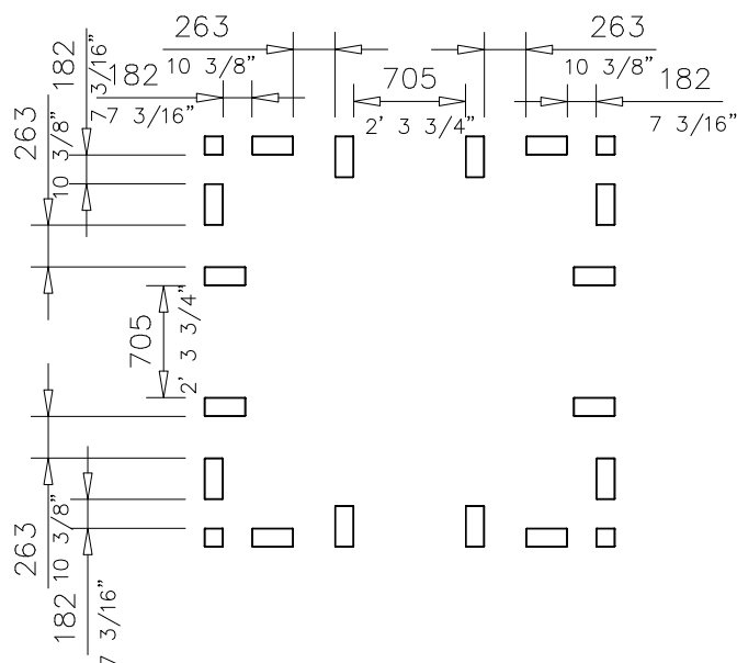
DET 34
