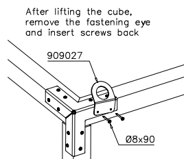
DET 33
