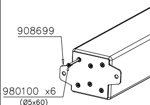
DET 23
