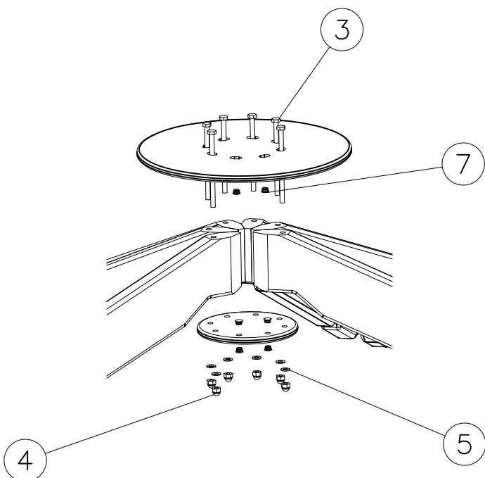
DET 1
