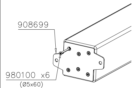
DET 6
