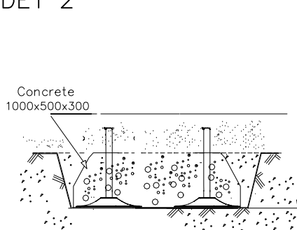
DET 2
