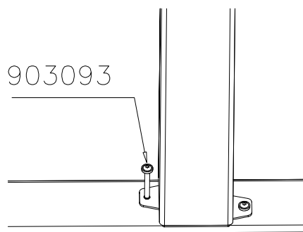
DET 7
