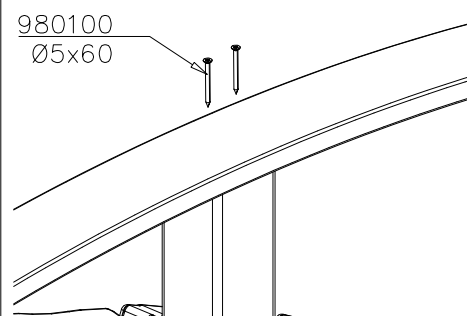
DET 3
