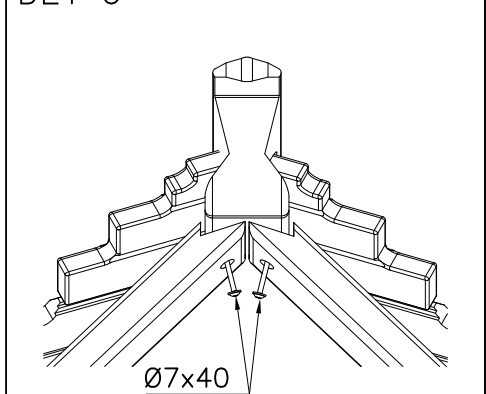
DET 6
