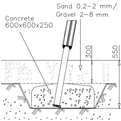
DET 4
