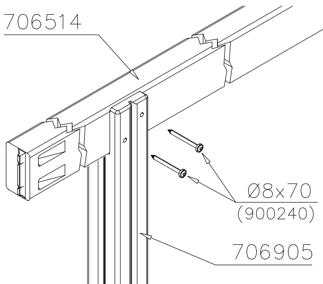
DET 12
