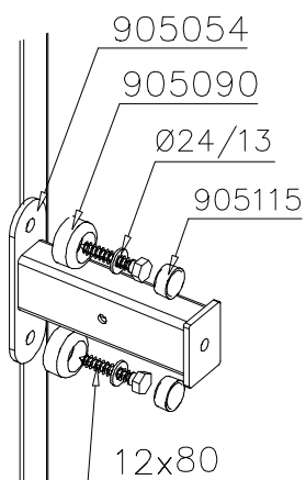
DET 1
