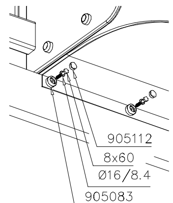
DET 3
