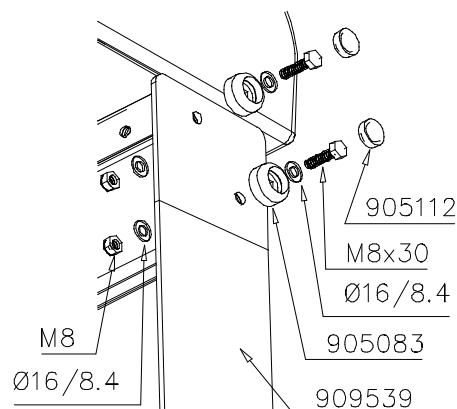
DET 2
