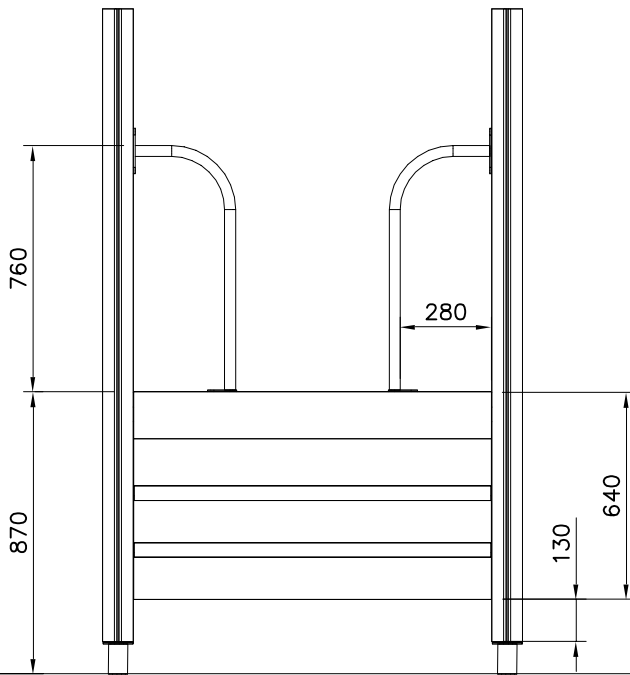
DET 2
