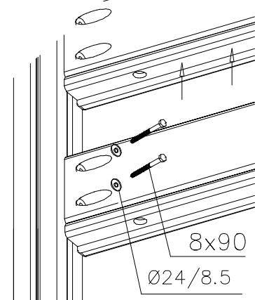
DET 1
