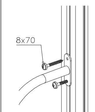
DET 2
