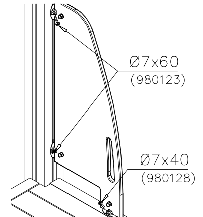
DET 3
