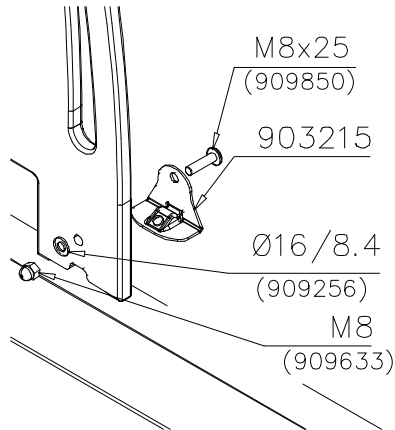
DET 2
