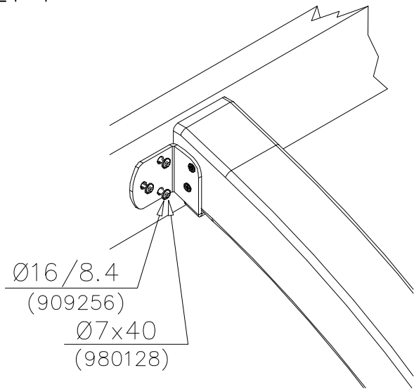
DET 4
