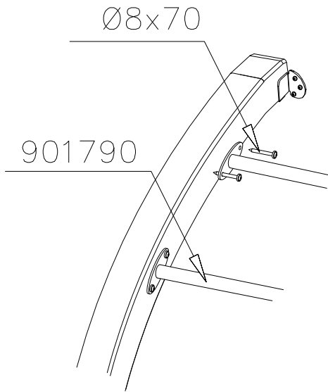
DET 1
