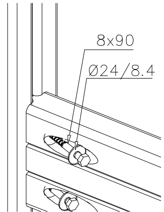
DET 3
