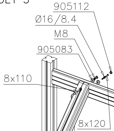
DET 5
