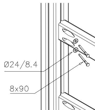
DET 6
