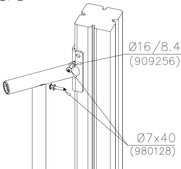
DET 4
