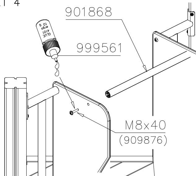
DET 4
